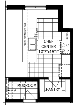
1 Chef Center
