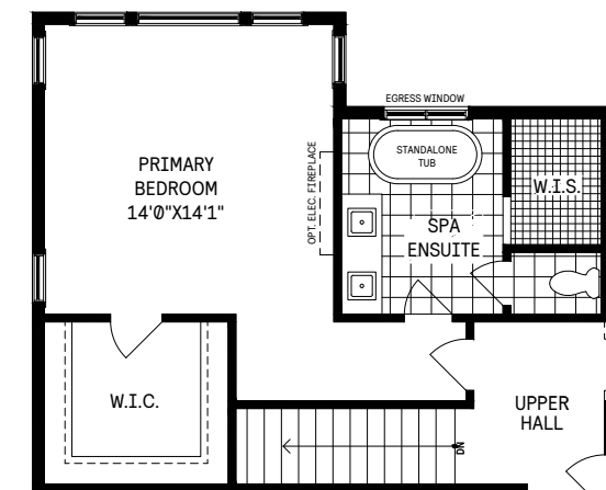
3 Spa Ensuite
