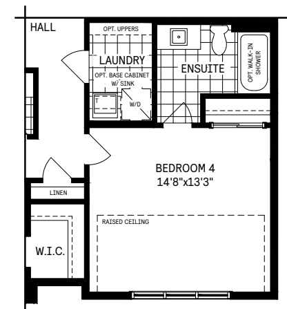
5 Bedroom 4 Ensuite
