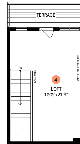
LOFT
