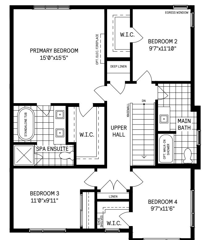
4 Spa Ensuite*
