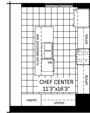
1 Chef Center
