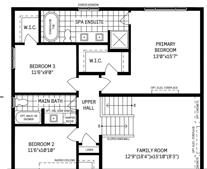
4 Spa Ensuite*
