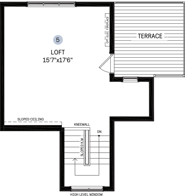
LOFT
