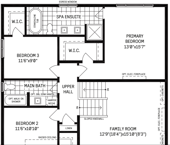
4 Spa Ensuite*
